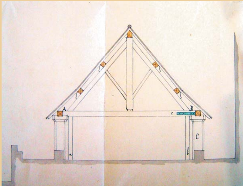
Coupe des halles couvertes dressée par l'architecte Dessalles en 1871.
